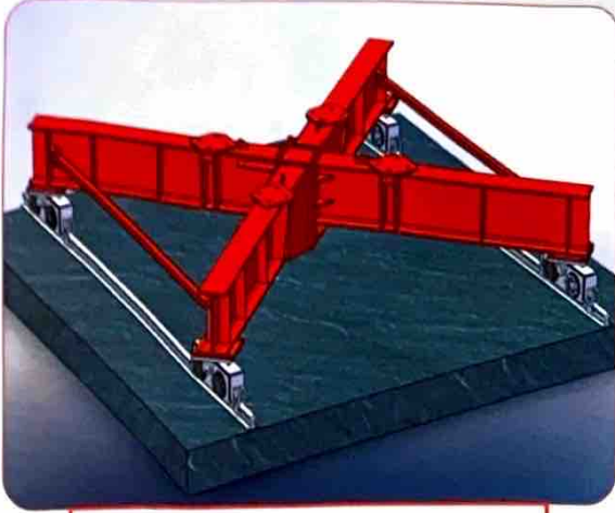
Yürüyüşlü Şase / Base With Bogies
