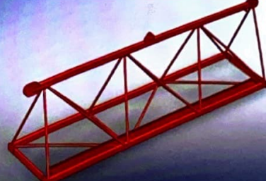
8 Numaralı BOM / JIB No 8
