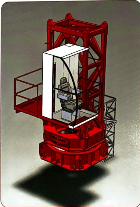
Dönüş Bölümü / Slewing Unit
